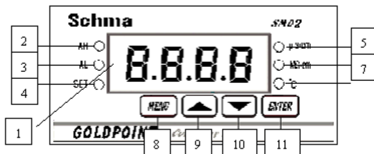
圖 4 儀表操作面板圖
