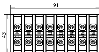
圖 2 儀表安裝孔開孔尺寸
