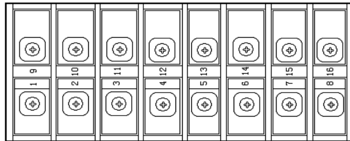
圖 5 儀錶端子圖
