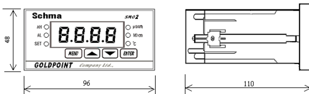
圖 1 儀表外形尺寸
